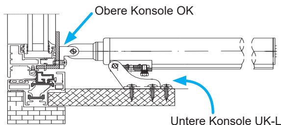
Abbildung 11: Klappflügel mit breiter Laibung
