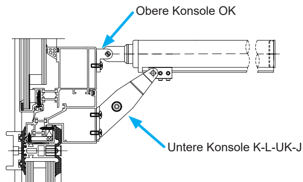
Abbildung 12: Bündiger Klappflügel
