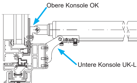
Abbildung 13: Klappflügel in Pfosten-/Riegelkonstruktion
