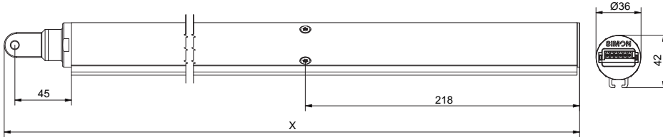
Abbildung 2: Abmessungen
