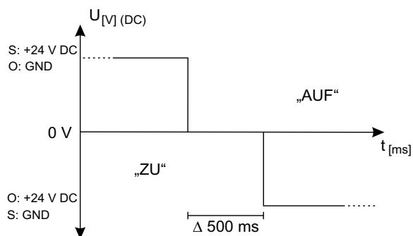
Abbildung 19: Null-Volt Bereich bei Fahrtrichtungsänderung
