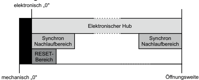
Abbildung 18: Hubverhalten
